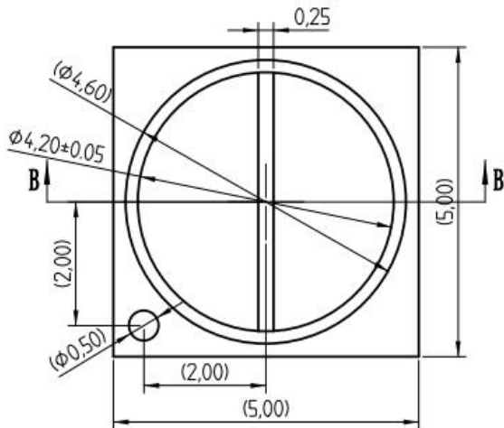
封装尺寸 Package Dimensions
